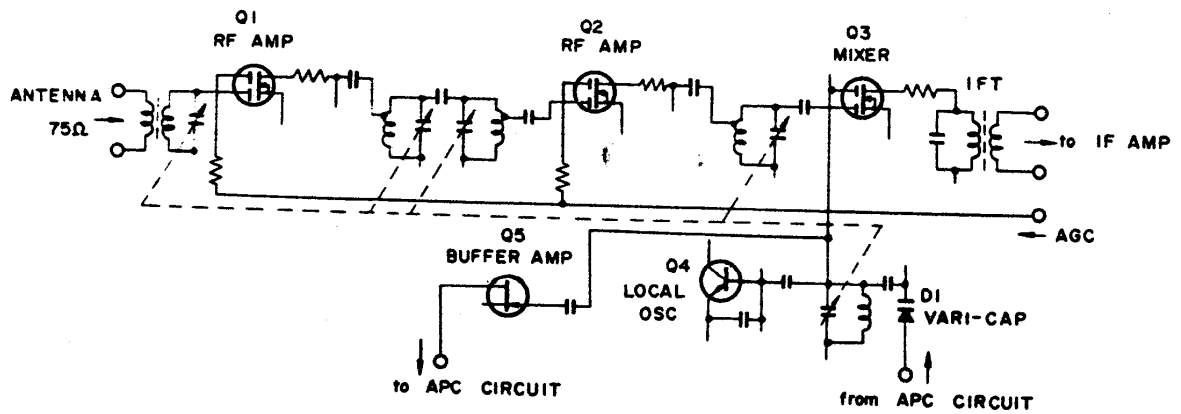
Fig. 4-1 FM front-end
