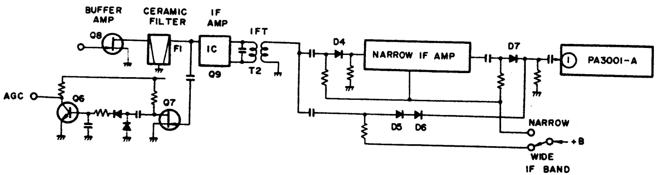
Fig. 4-2 FM IF amplifier
